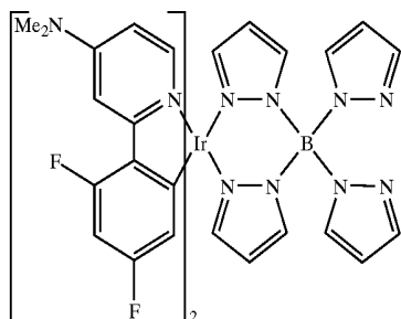
(dmafppy)_2Ir(pz_2Bpz_2)
